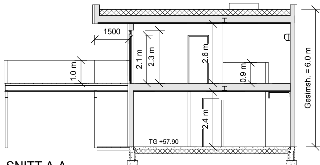
SNITT A-A
